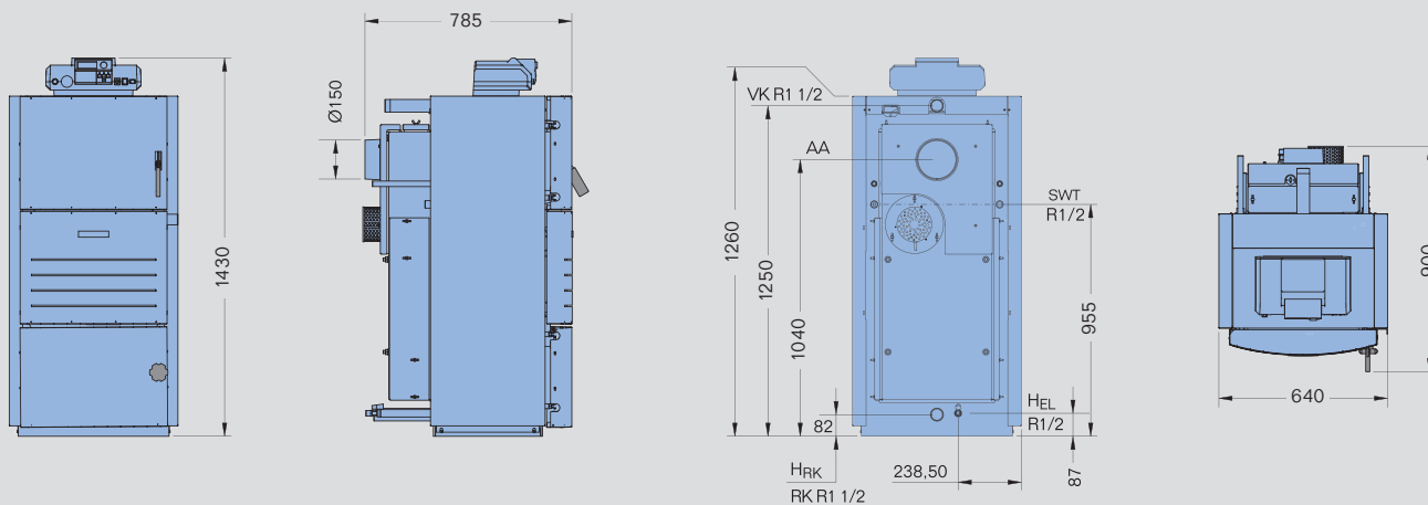
Rozmery a pripojenia Logano S161 - 18
