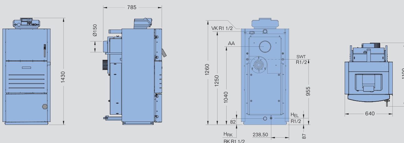
Rozmery a pripojenia Logano S161 - 24
