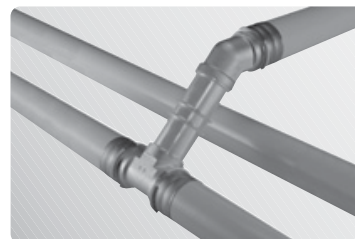
Použitie komponentu „spacer“ pre odbočku vetvy potrubia
